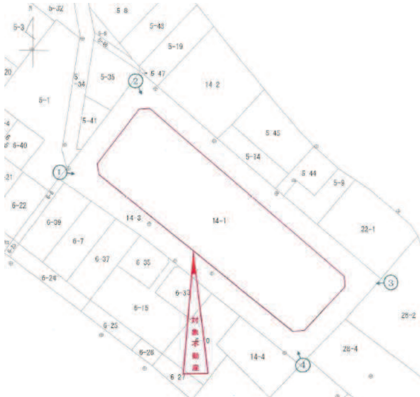
整理図
