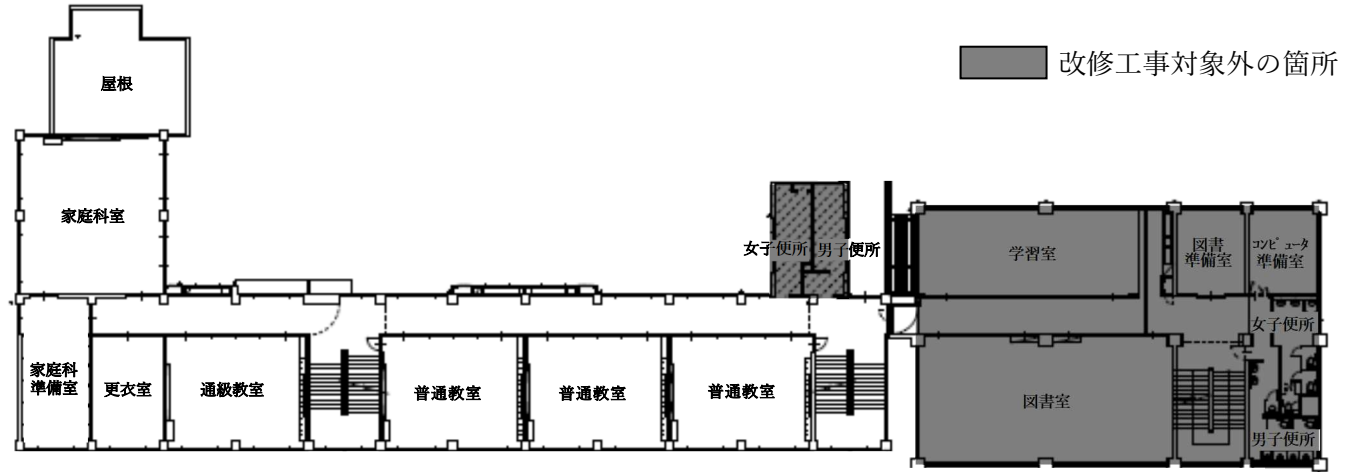
南校舎 2階平面図 改修前
