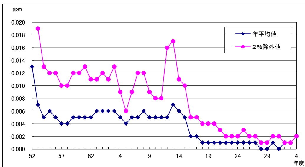
二酸化硫黄の経年変化 (一般環境大気測定局 豊川市役所)
