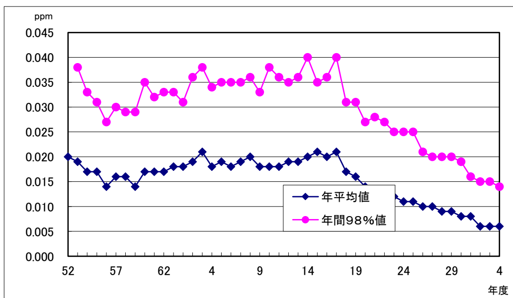
二酸化窒素の経年変化(一般環境大気測定局 豊川市役所)
