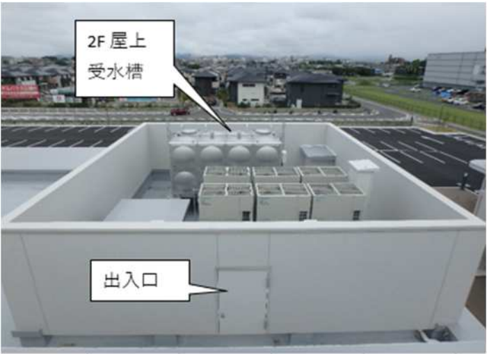
2 F 屋上受水槽（8.0 m³）
