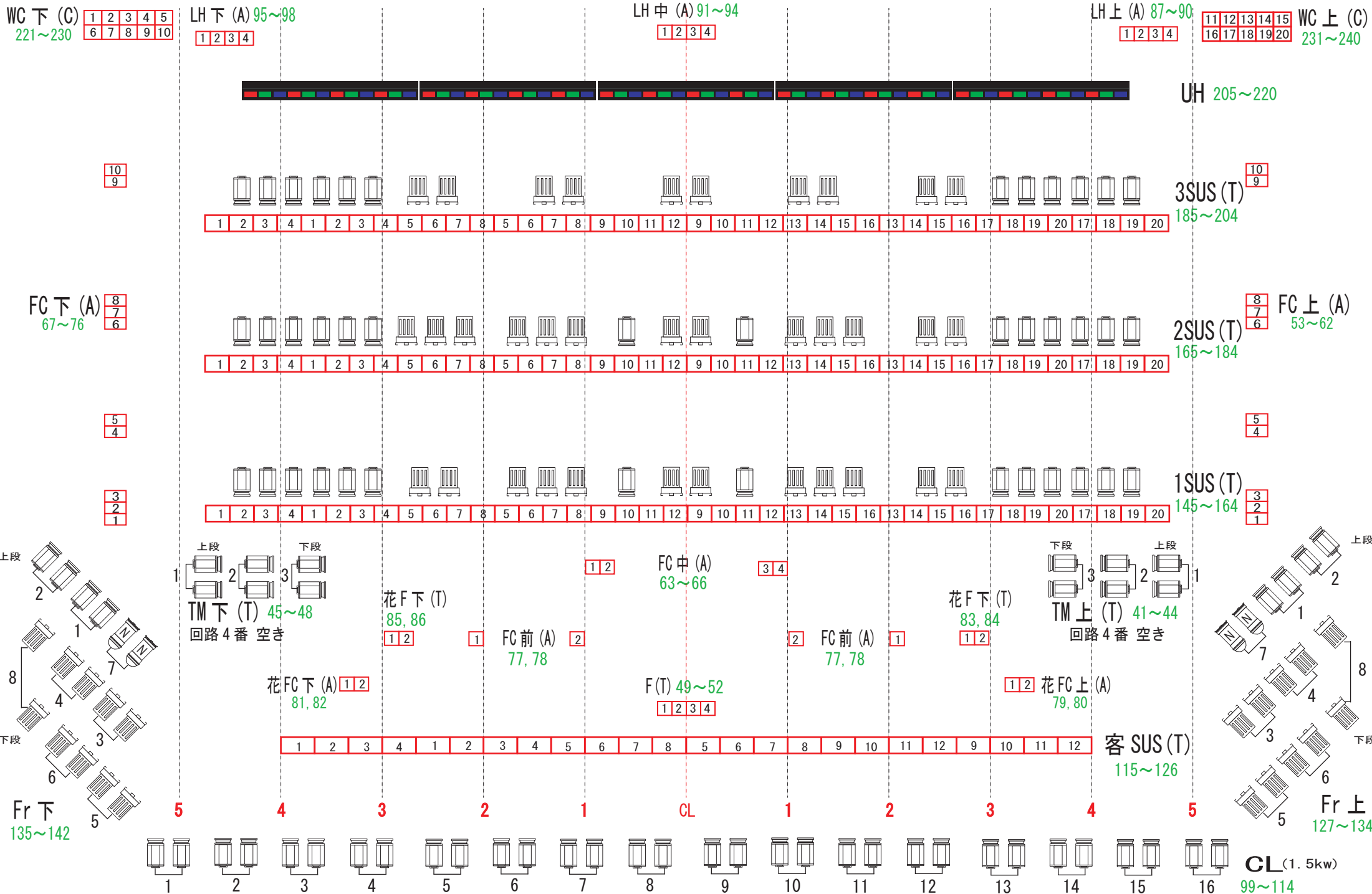
豊川市文化会館 基本吊り込み図
