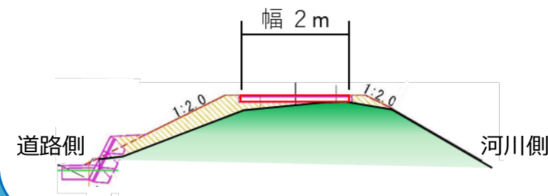
【参考断面図 (左岸)】
