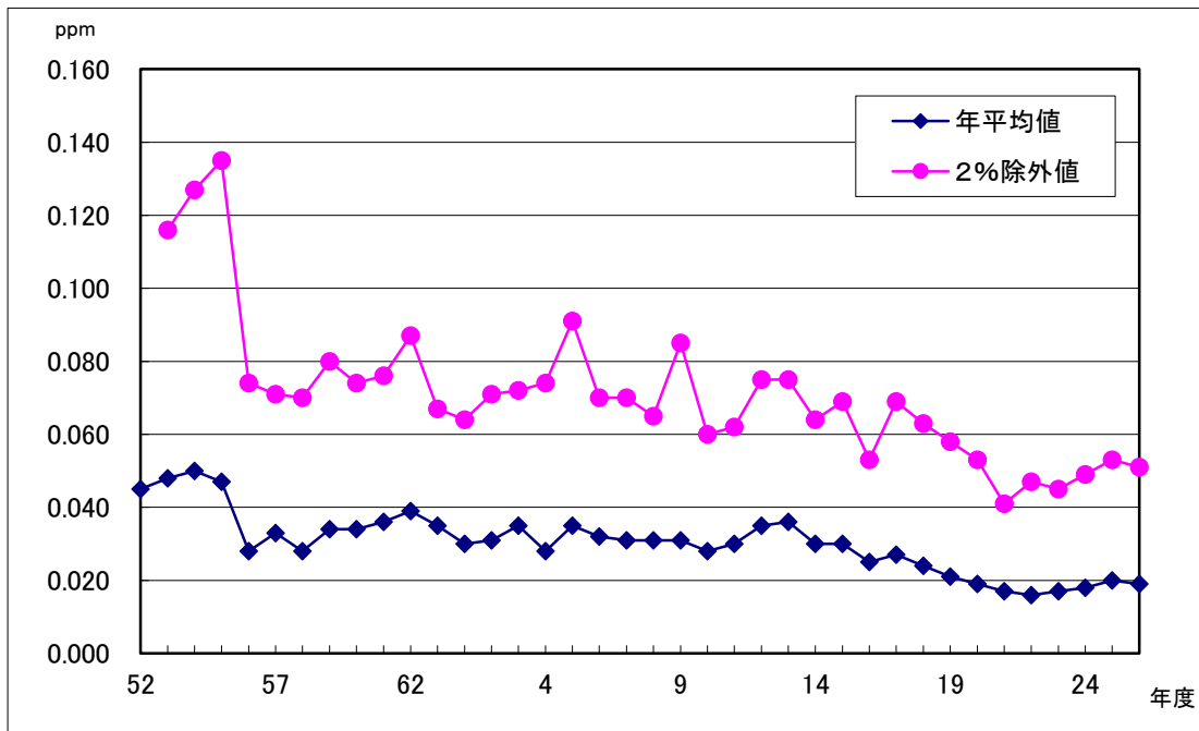
浮遊粒子状物質の経年変化(一般環境大気測定局 豊川市役所)
