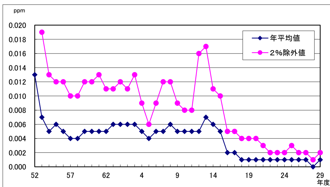
二酸化硫黄の経年変化（一般環境大気測定局 豊川市役所）
