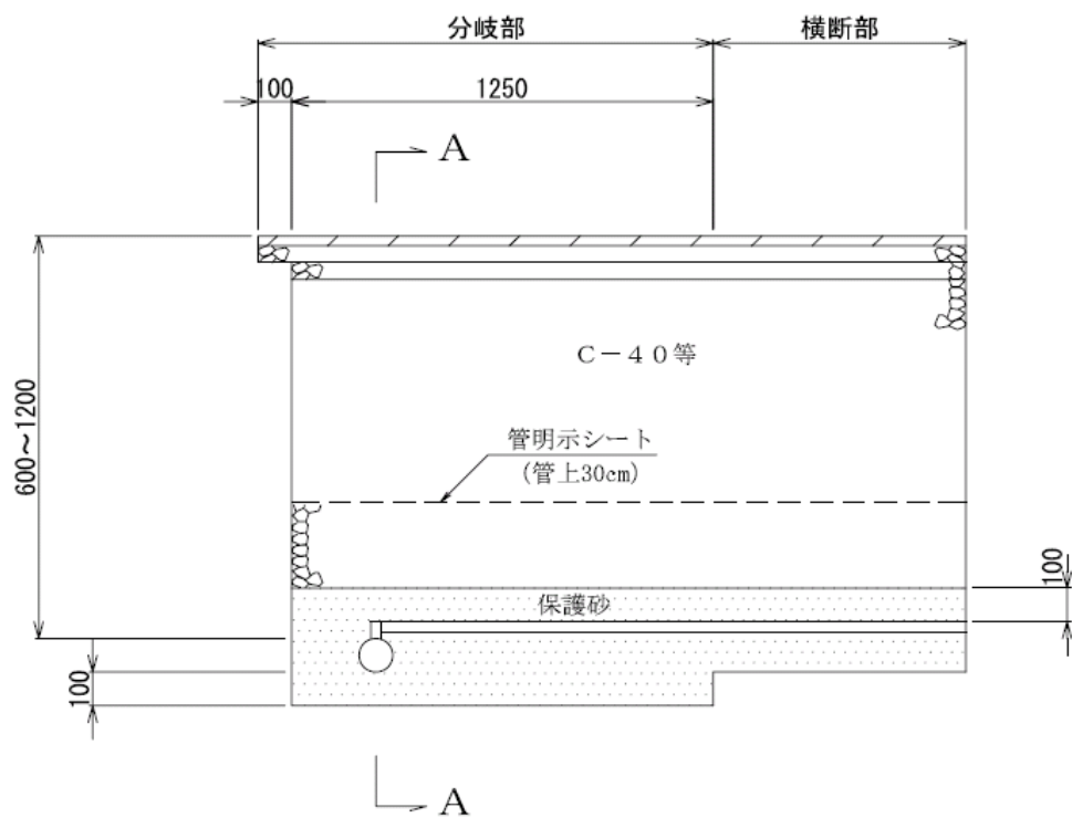
断面図
