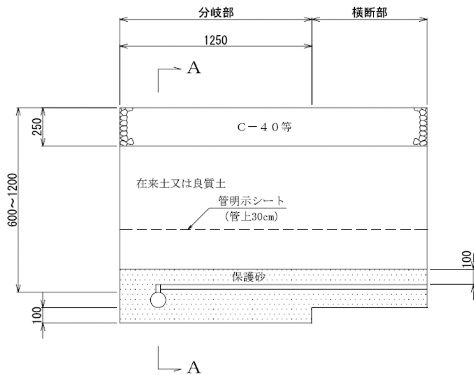
断面図
