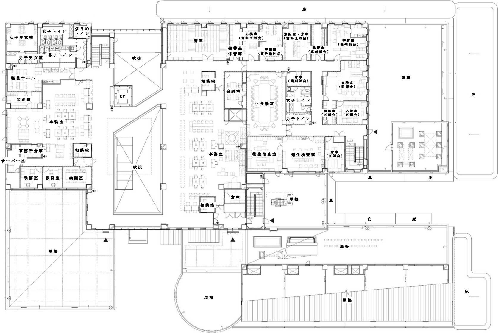
2 階平面図
