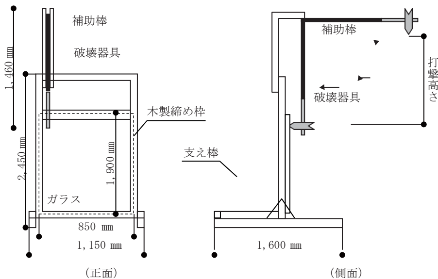
図1 本体
