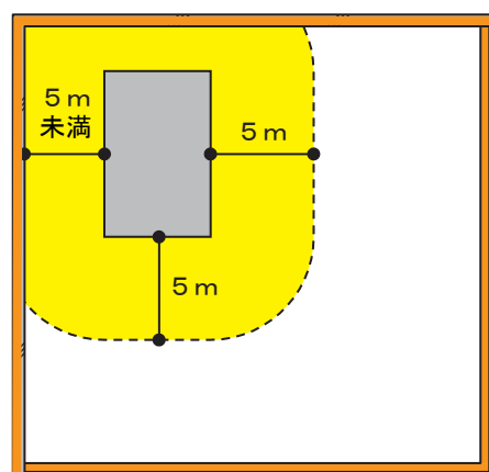
○不燃材料で造られた壁がある場合
