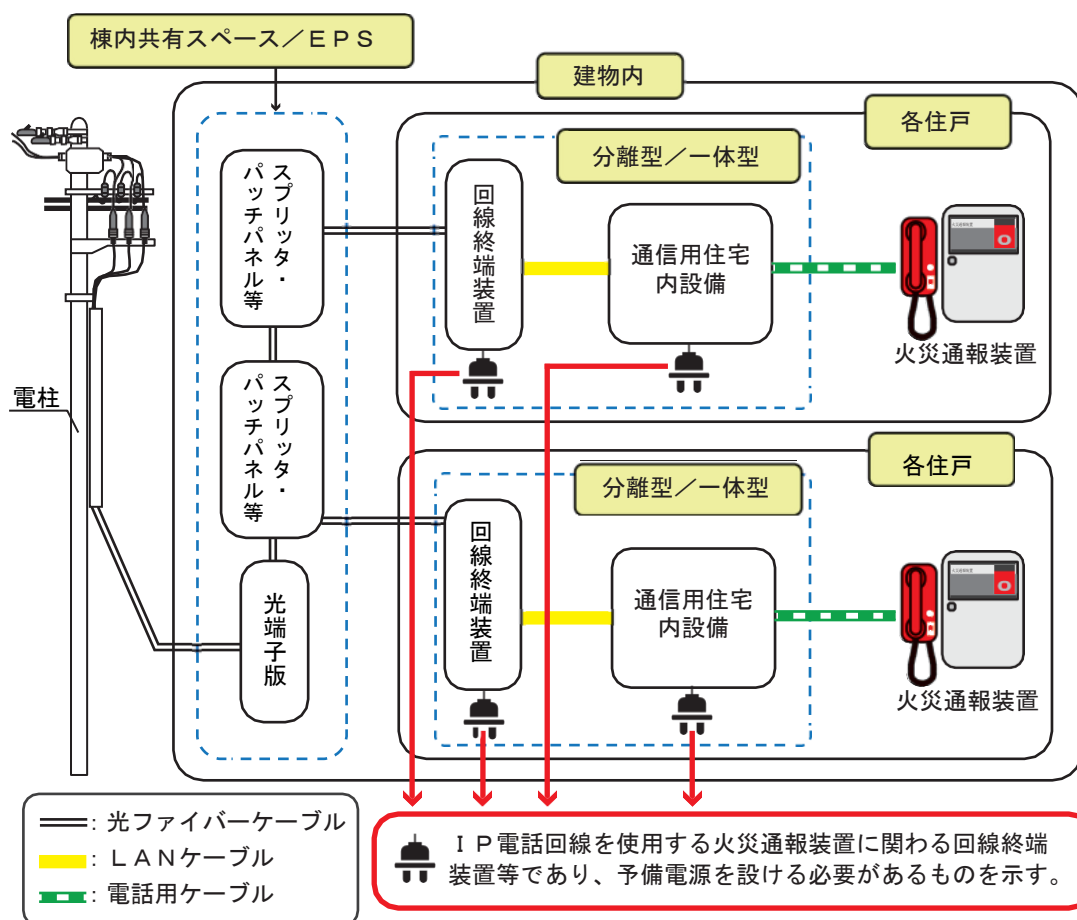
【光配線方式】
