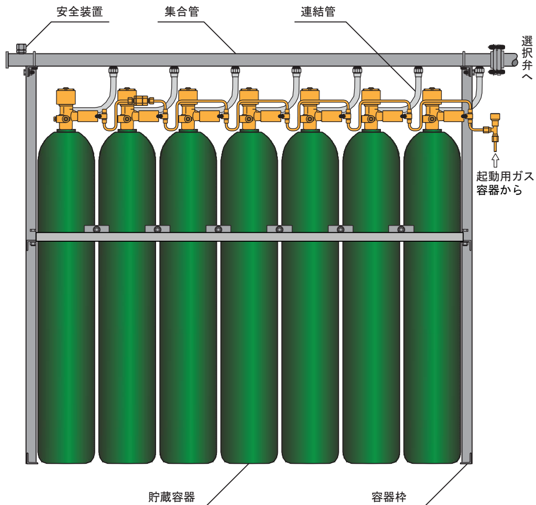
（参考）高圧式貯蔵容器周りの構成例
