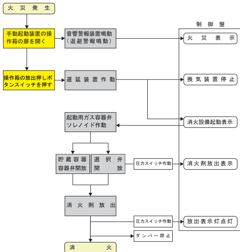
（参考）手動式の場合のフロー
