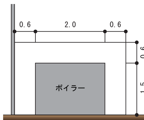
(立面図)
