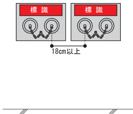
（頭部回転型送水口の場合）
