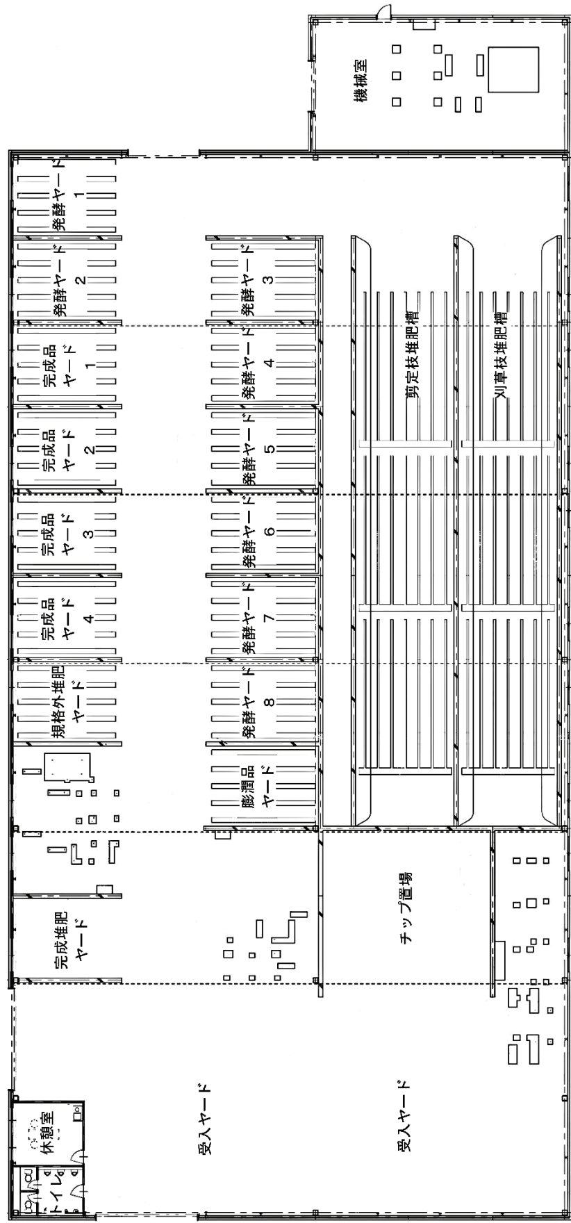
刈り草・剪定枝破碎堆肥化施設平面図
