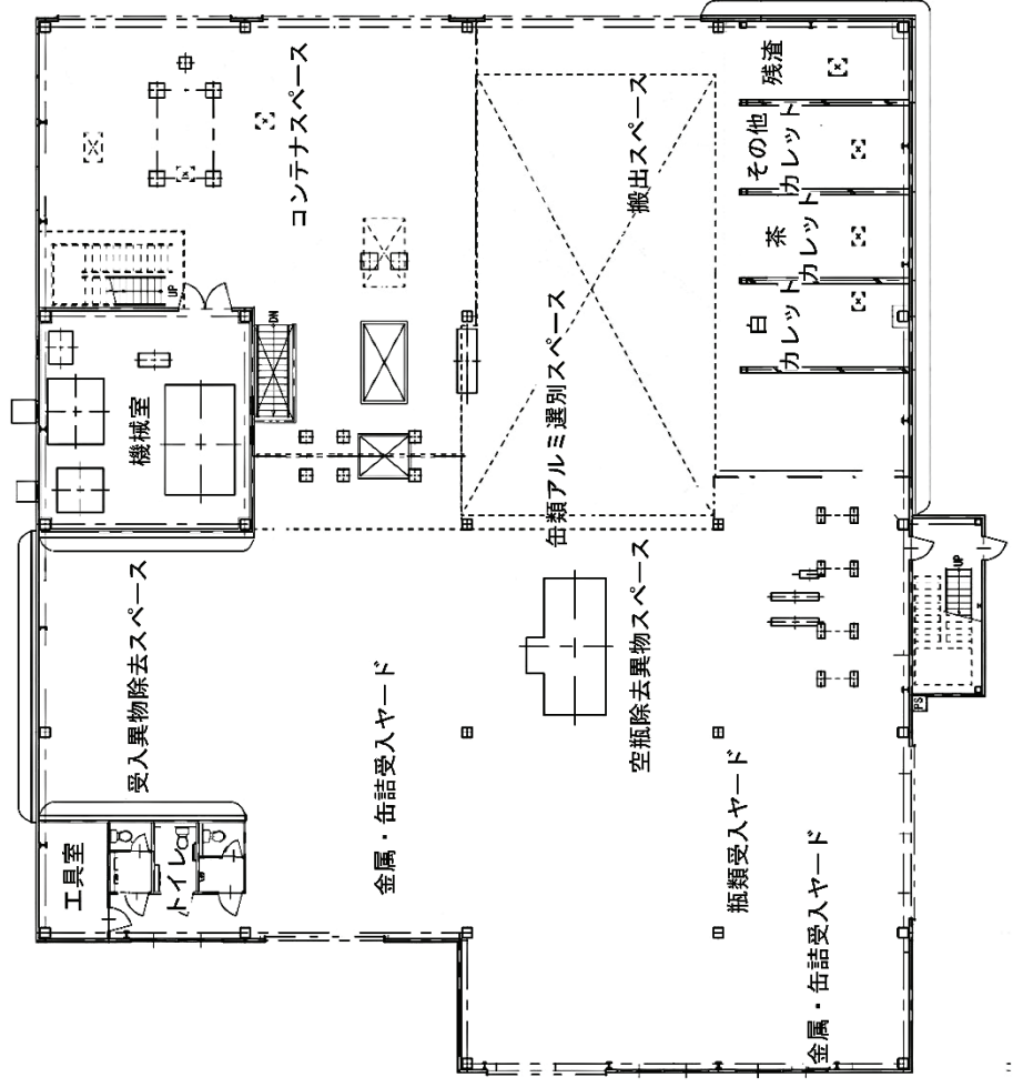
1階平面図
