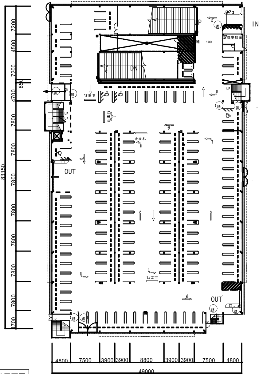
1階平面図
