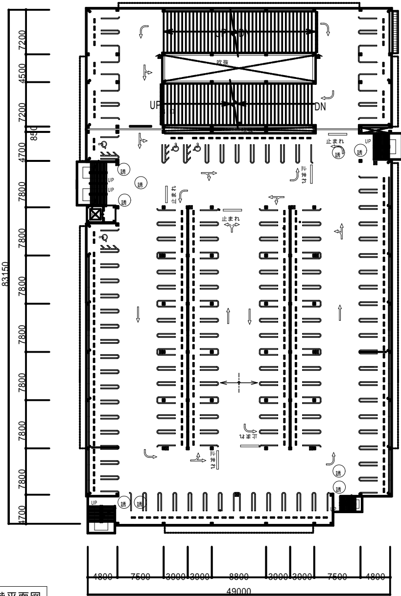
2階平面図
