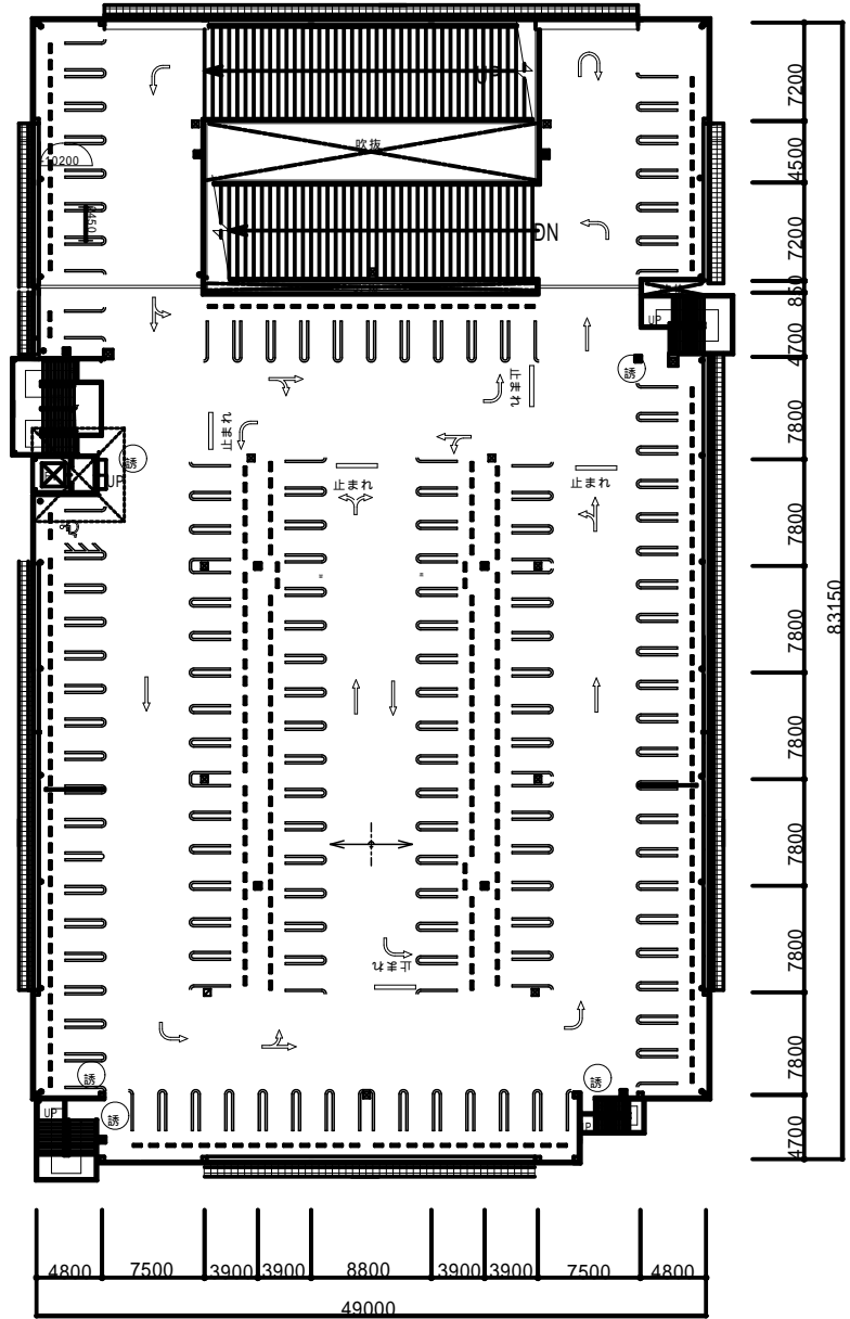
P H 階部分平面図
